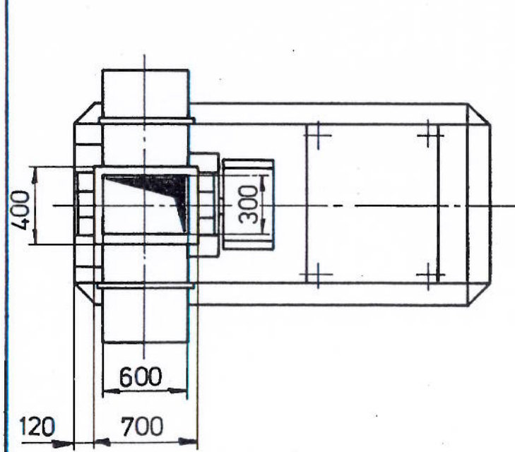
Molino a martelli
